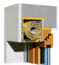
Vorbau-Einputz-Rollladen FR 41
