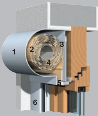
Halbrund-Sicherheits-Rollladen FR 24
