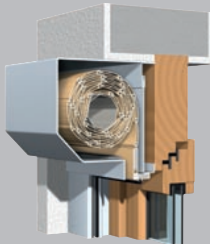
Sicherheits-Rollladen mit abgeschrägtem Kasten FR 23
