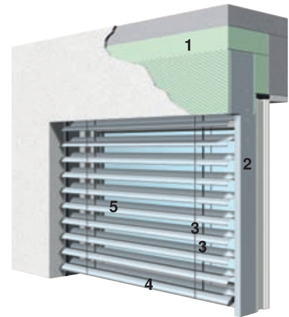
Fenster-System-Raffstore, FSR 3 mit Abdunkelungs-Raffstore E 93 A6
